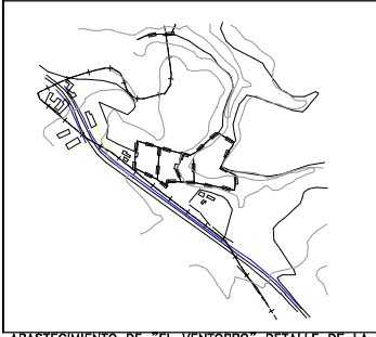
ABASTECIMIENTO DE "EL VENTORRO" DETALLE DE LA DISTRIBUCION
